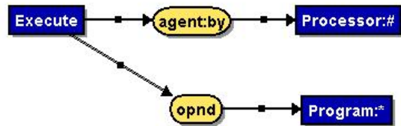
Figura 12. Representaciones textual y gráfica en grafos conceptuales de la frase “Un programa es ejecutado por el procesador”.
