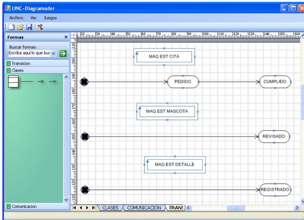
Figura 32. Diagramas de máquina de estados resultantes en UNC-Diagramador para la Clínica Veterinaria.
