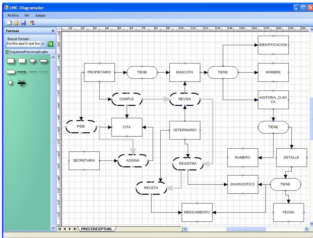
Figura 29. Imagen del Esquema Preconceptual resultante para la Clínica Veterinaria.
