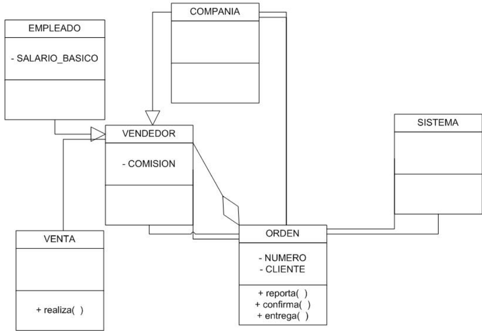
Figura 39. Diagrama de clases resultante del Esquema Preconceptual de la Figura 38.
